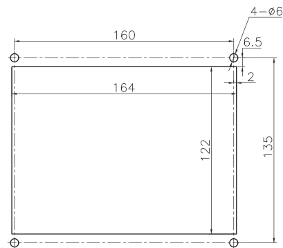
매립치수
