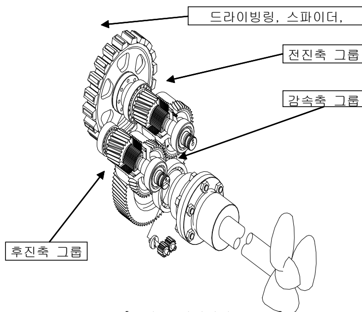
[그림-1 마린기어 구조도]
