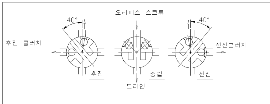
[그림-5 변환밸브 구조] -(그림6의 단면 A-A)
