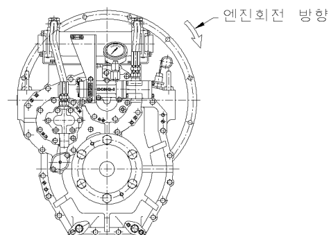
[역회전 엔진]
