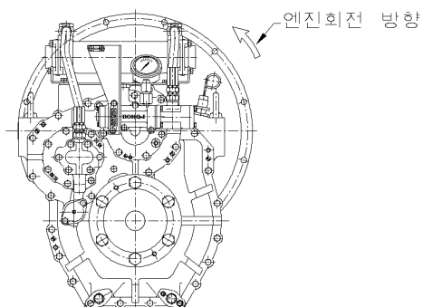
[정회전 엔진]
