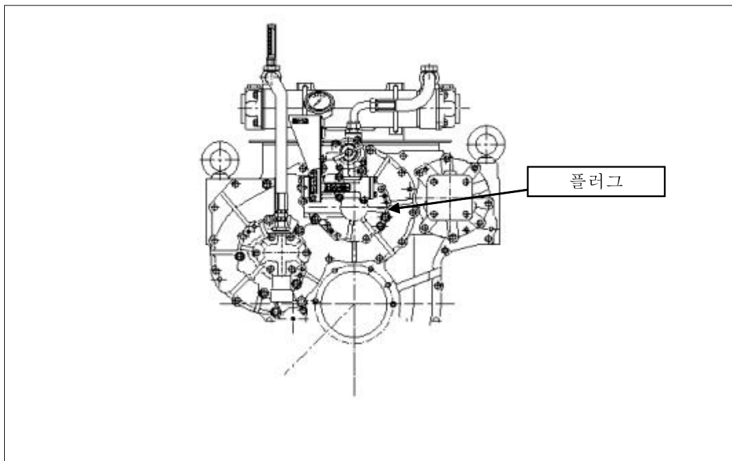
[그림-7 긴급스크류 위치]
