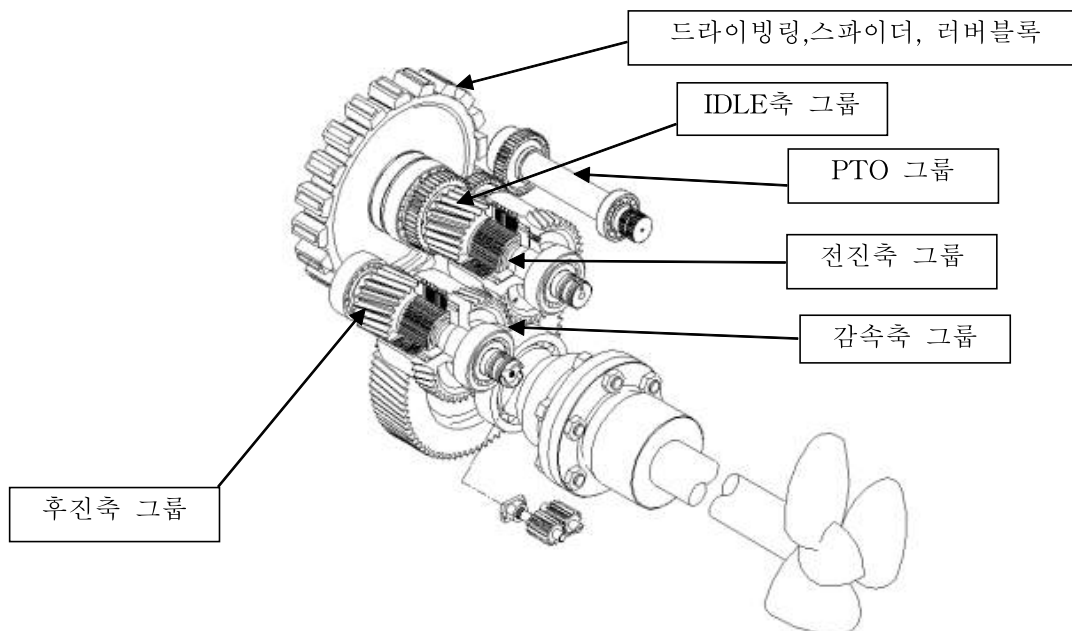
[그림-1 마린기어 구조도]
