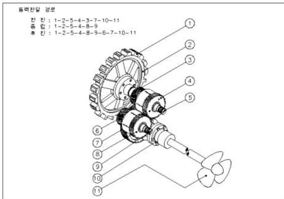
[그림-2 동력전달계통]
