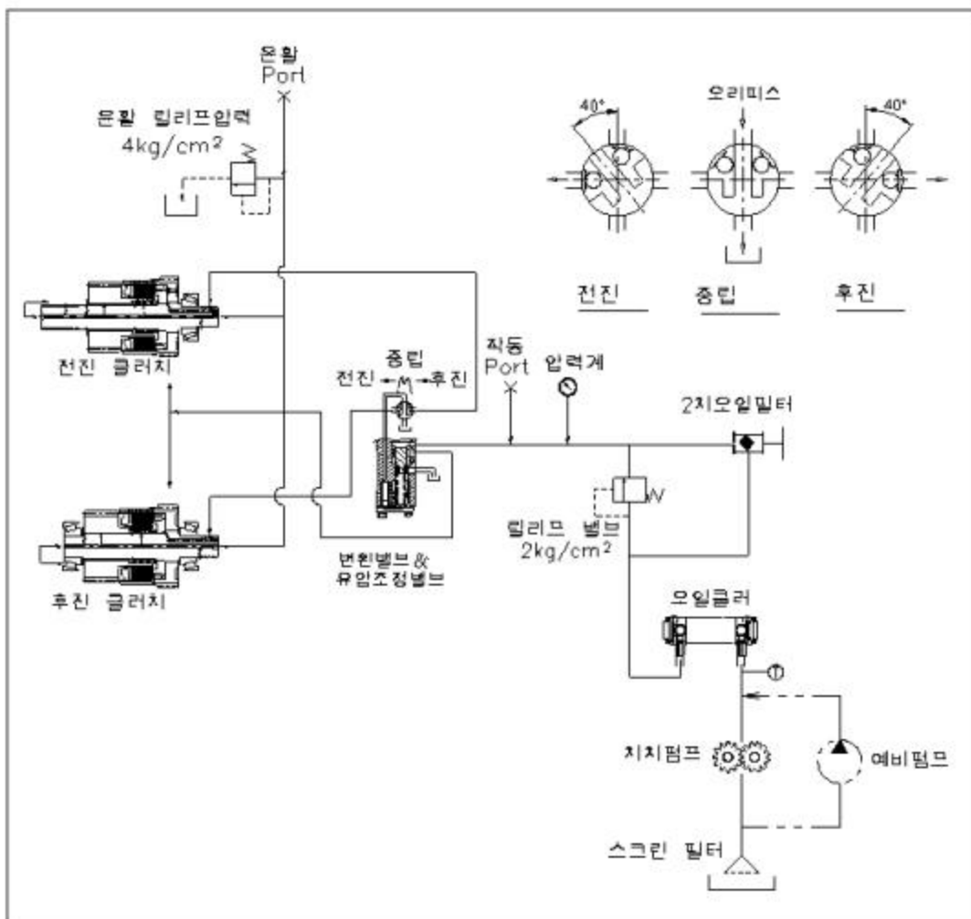
[그림-4 유압회로도]
